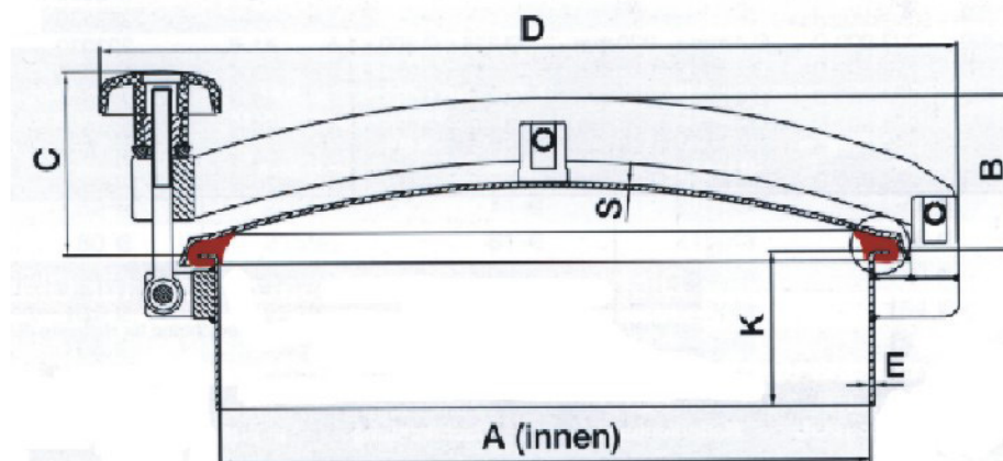
Dichtungsdetail NW 200-800
